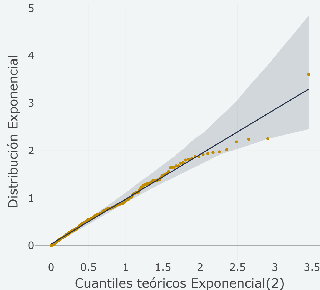
QQ-plot (exponencial)
